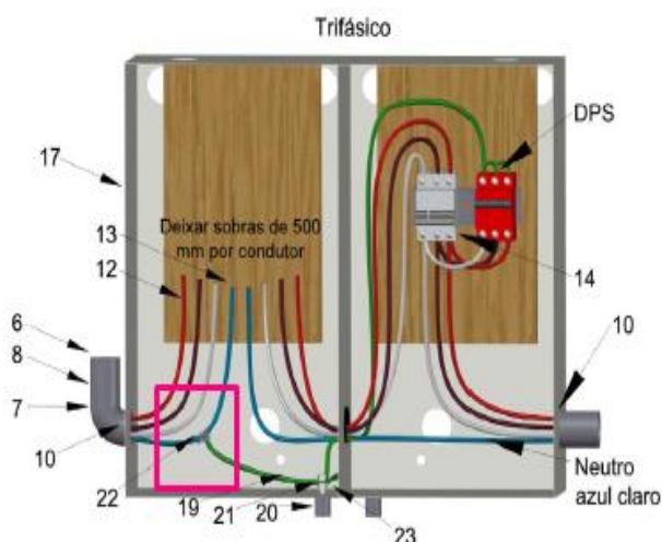
Figura 3: Equipotencialização entre Condutores de Neutro e Proteção, conforme GED 13
