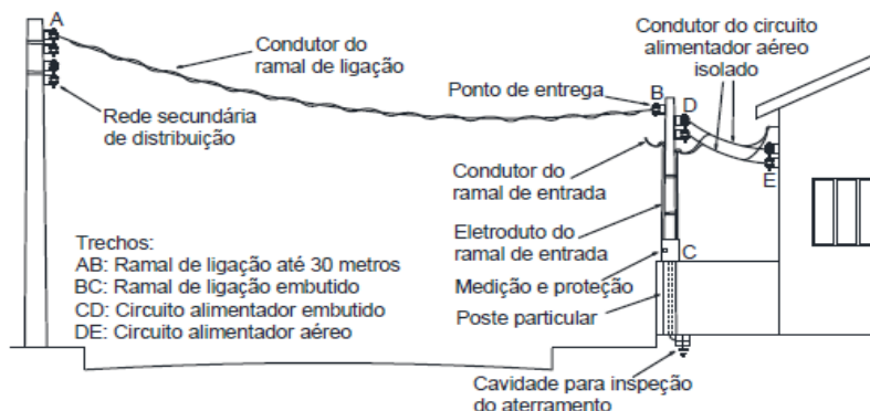
Figura 1: Componentes entrada de serviço - GED13
